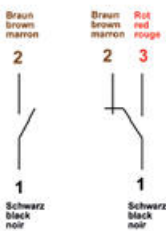
Kopplingsbild transmitter
