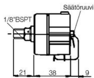
Modell 6742
