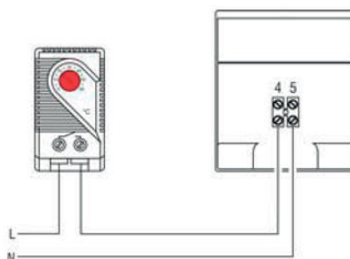
Termostat KTO011 Heater CS(L) 028
