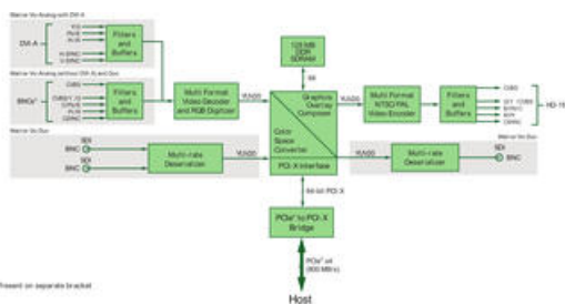
Blockdiagram - Matrox Vio familj
