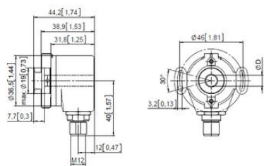
5 - Statorkoppling
