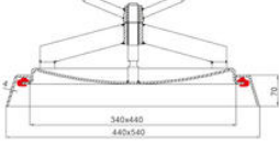
Dæksel med presset karm
